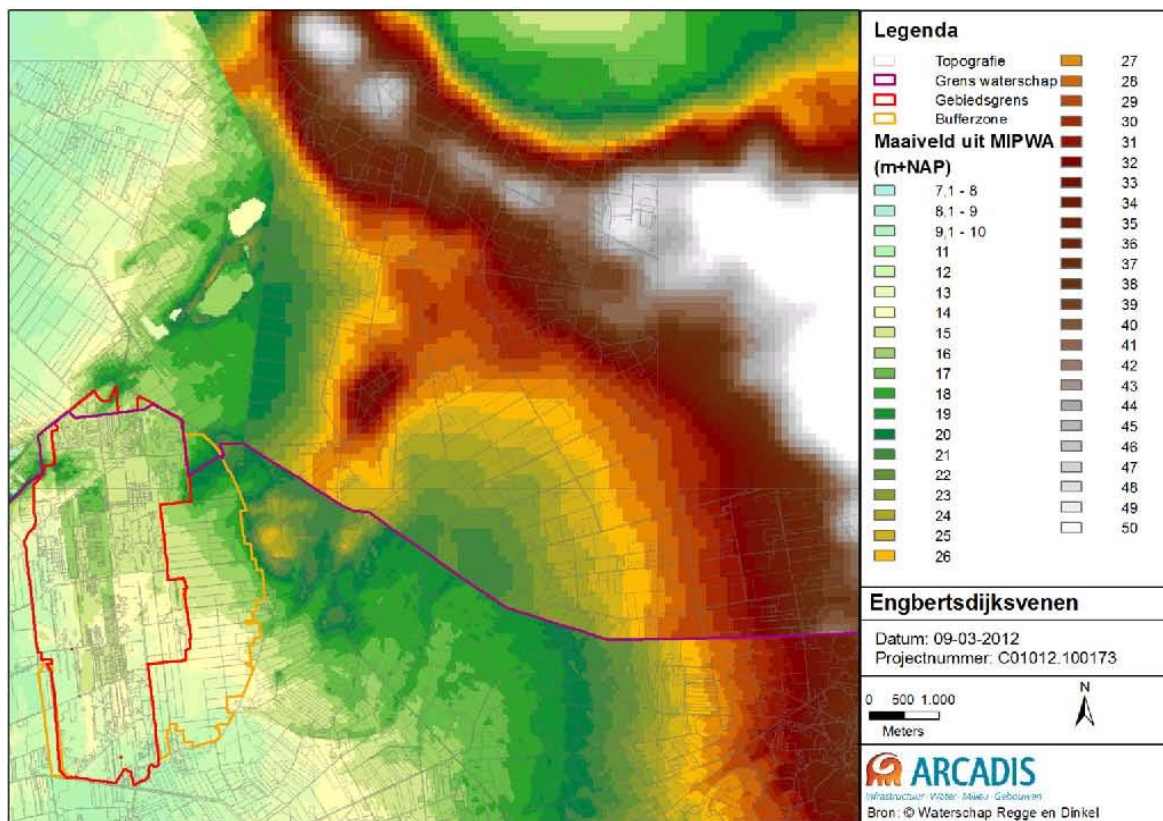
Figuur 3.2. Maaiveldhoogtekaart van de omgeving van Engbertsdijkerven. De schijnbare verschillen in hoogteligging op de grens van Duitsland en Nederland bestaan in werkelijkheid niet. Het Duitse deel is waarschijnlijk circa 2 meter te laag weergegeven.
