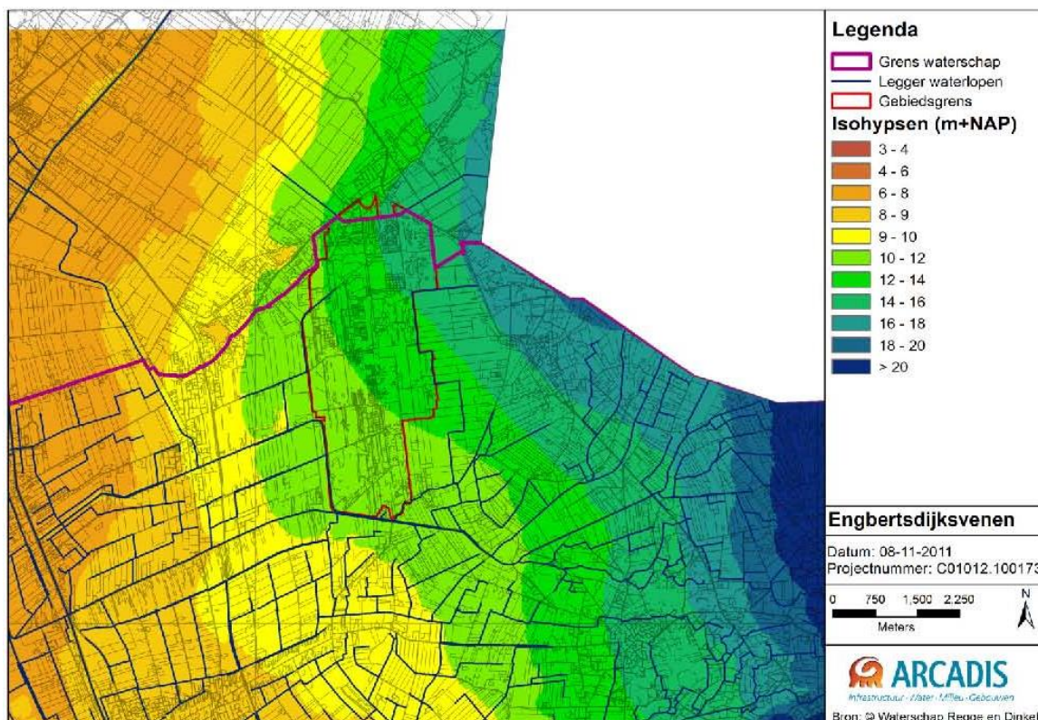
Figuur 3.11. Isohypsens bij een gemiddelde situatie in de omgeving van Engbertsdijkerven.
