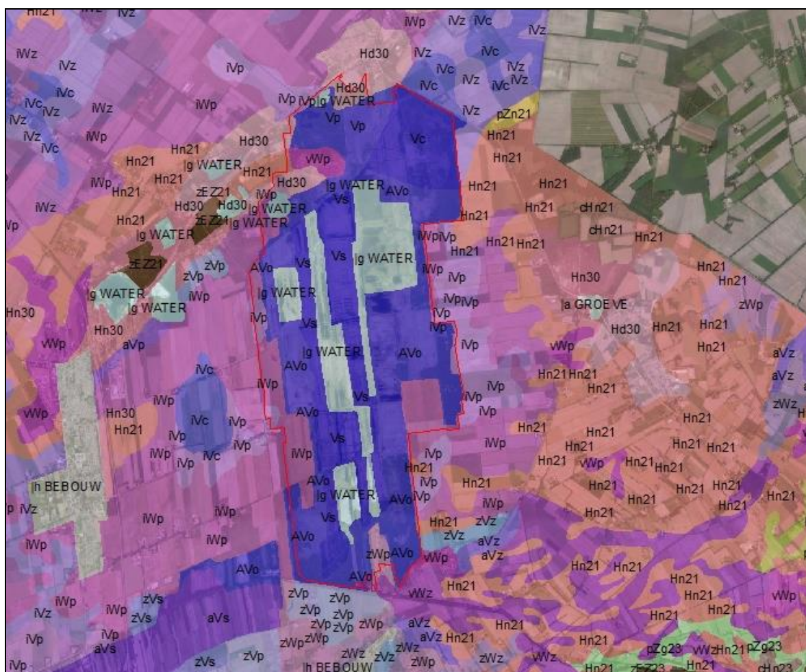
Figuur 3.7 Bodemkaart 1:50.000. Bron: Alterra
