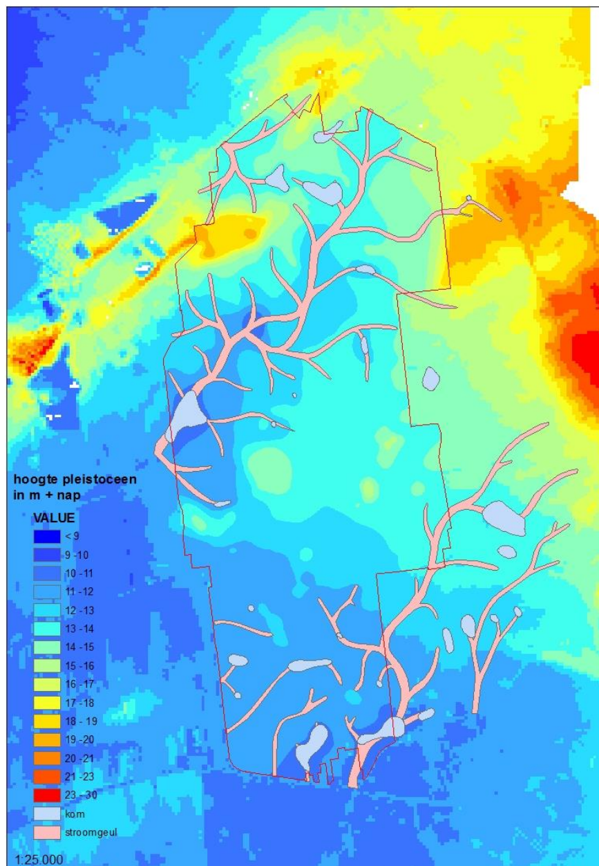
Figuur 3.4. Maaiveldhoogtekaart van de zandondergrond in het Natura 2000-gebied Engbertsdijkerven, ingebed in de maaiveldhoogtekaart van de omgeving. Met kleuren zijn de hoogten aangegeven in m t.o.v. NAP. Tevens zijn stroomgeulen en kommen aangegeven, naar een reconstructie van Maris en Roelofsen. Een midden tussen de 2 grotere stroomgeulen aangegeven derde stroomgeul is verwijderd omdat die op een te hoog niveau in het landschap zou liggen.
